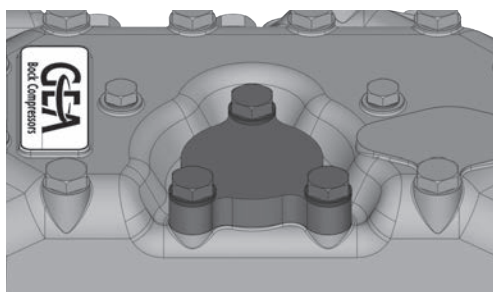
Состояние при поставке 1 (с завода): Рис. 30 Крышка цилиндра подготовлена для регуляторов мощности.
