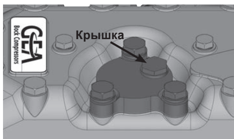
Рис. 31 Состояние при поставке 2 (с завода): Регулятор производительности, смонтирован с кожухом (защита от повреждений при транспортировке).
